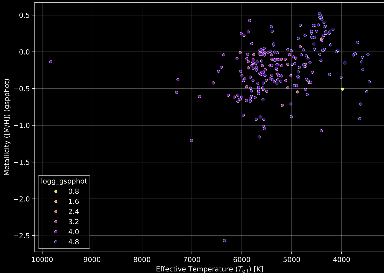
APOGEE DR17 Field: [247+62_btx] Stellar Population Parameters (n= 218)
